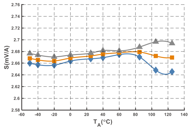
图 15 灵敏度曲线 (@I PN = 1500 A)
