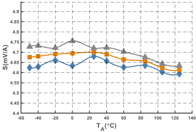
图 12 灵敏度曲线 (@I PN = 850 A)
