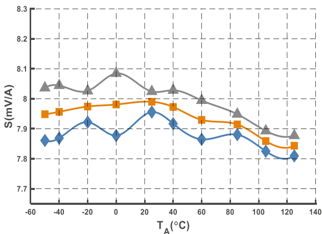
图10 灵敏度曲线 (@ I_{PN} = 500 \text{ A} )
