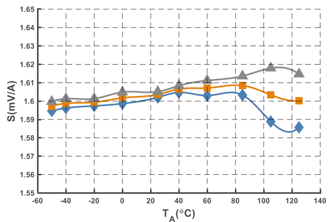
图 17 灵敏度曲线 (@I PN = 2500 A)
