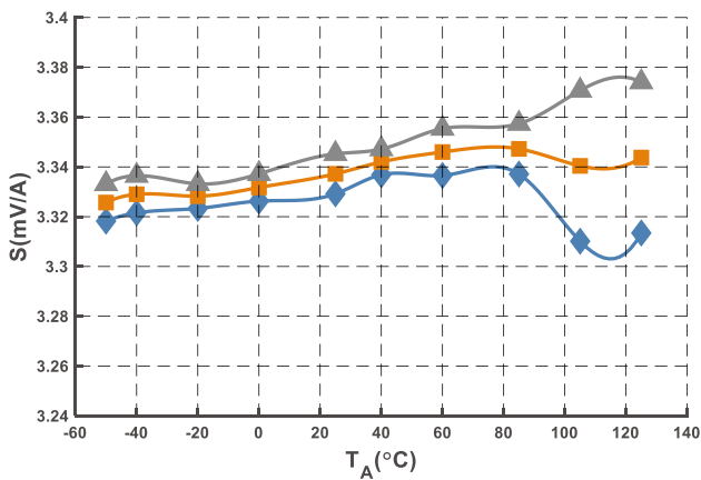
图 14 灵敏度曲线 (@I PN = 1200 A)
