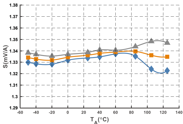
图 18 灵敏度曲线 (@I PN = 3000 A)
