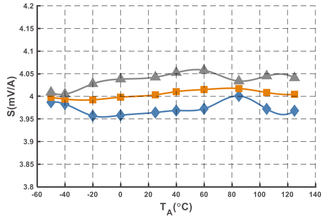
图 13 灵敏度曲线 (@I PN = 1000 A)
