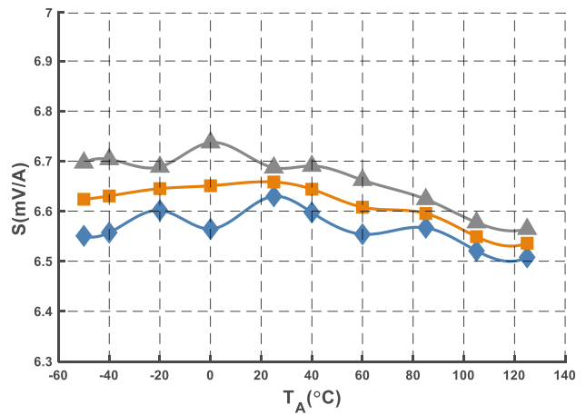
图11 灵敏度曲线 (@ I_{PN} = 600 \text{ A} )
