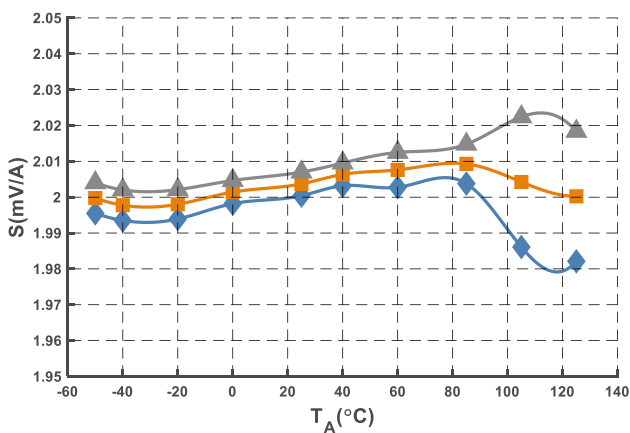
图 16 灵敏度曲线 (@I PN = 2000 A)
