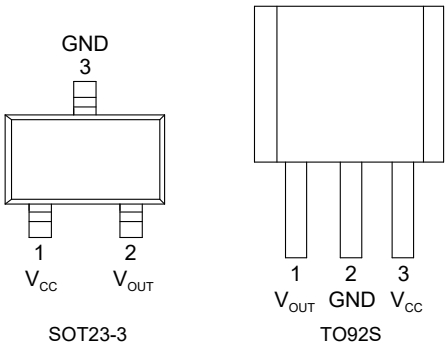
图 4 引脚定义
