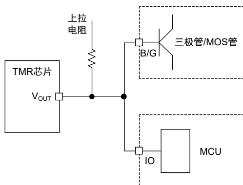
图 8 驱动功率负载的应用电路
