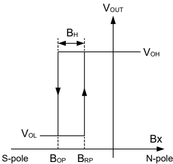
图 3-1 芯片磁场响应曲线 (SOT23-3)
