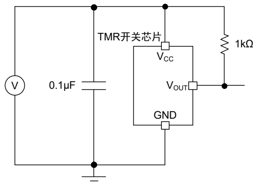
图 7 滤波电容用以降低供电噪音
