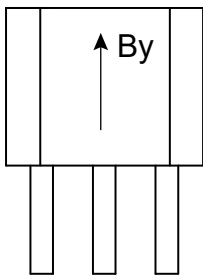
图 2-3 芯片敏感轴向图 (TO92S 侧视图)
