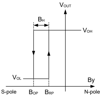
图 3-2 芯片磁场响应曲线 (TO92S)
