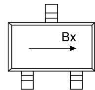
图 2-2 芯片敏感轴向图 (SOT23-3 俯视图)
