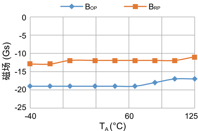
图 6 工作点、释放点和工作温度的关系 ( V_{CC} = 3\text{ V} )
