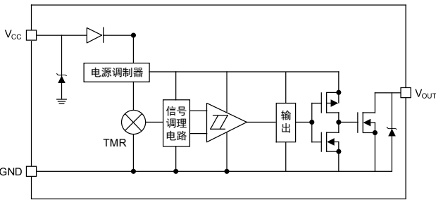
图 1 芯片内部原理框图
