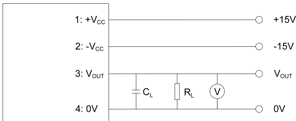
图 16 电气接口接线图
