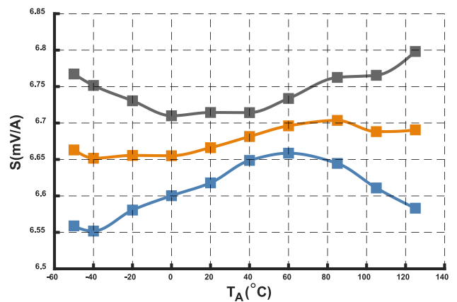
图 14 灵敏度曲线 (@ I_{PN} = 600\text{ A} )
