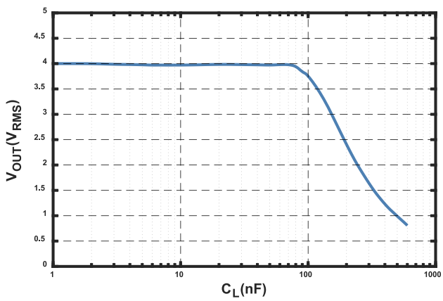
图 3 负载电容特性曲线 (@ I_P = I_{PN} )
