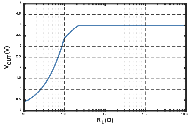
图 2 负载电阻特性曲线 (@ I_P = I_{PN} )
