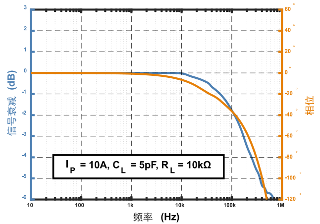
图 4 频响特性曲线
