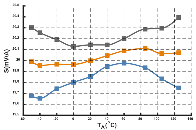
图 10 灵敏度曲线 (@ I_{PN} = 200\text{ A} )
