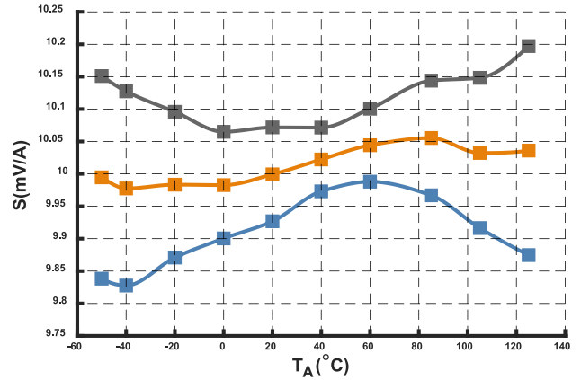
图 12 灵敏度曲线 (@ I_{PN} = 400\text{ A} )
