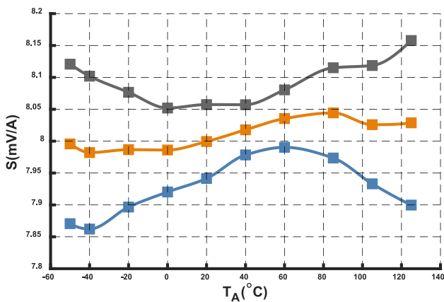
图 13 灵敏度曲线 (@ I_{PN} = 500\text{ A} )
