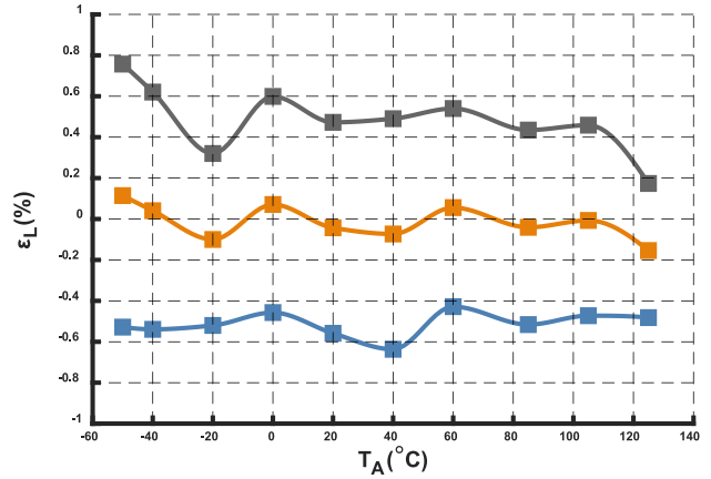
图7 线性度曲线
