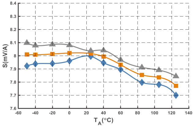
图 12 灵敏度曲线 (@I PN = 500 A)
