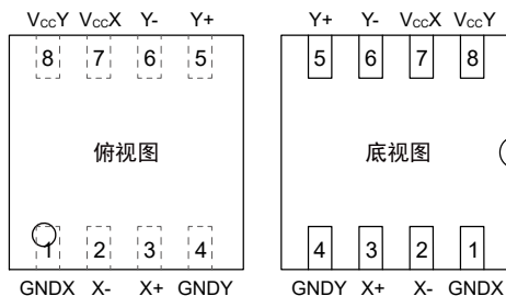
图 4 引脚定义 (LGA8L)
