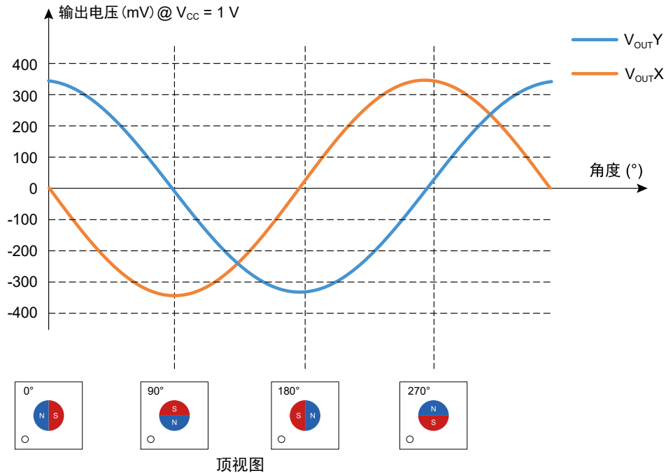
图 5 TMR3005 输出信号与磁铁关系示意图
