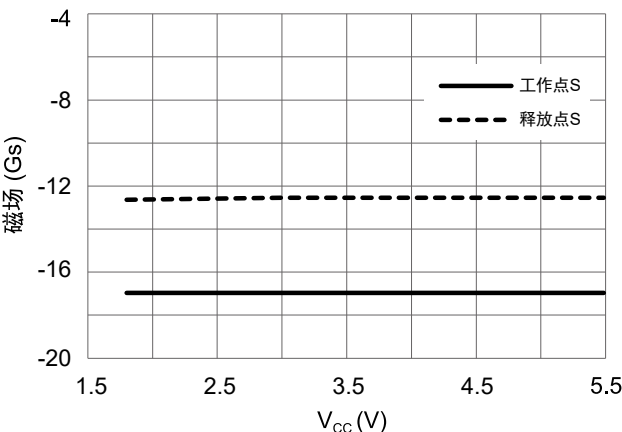
图 6 工作点、释放点和供电电压的关系 ( T_A = 25\text{ °C} )
