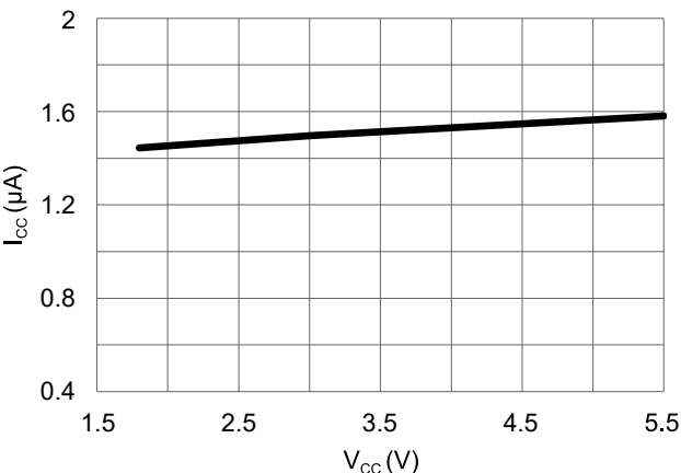
图 5 工作电流和供电电压的关系 ( T_A = 25\text{ °C} )
