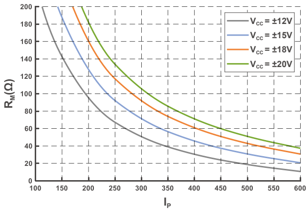
图 3 测量电阻 (@ T_A = 70\text{ }^\circ\text{C} )
