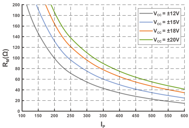
图 5 测量电阻 (@ T_A = 25\text{ }^\circ\text{C} )
