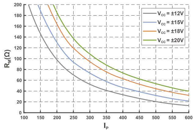
图 4 测量电阻 (@ T_A = 50\text{ }^\circ\text{C} )
