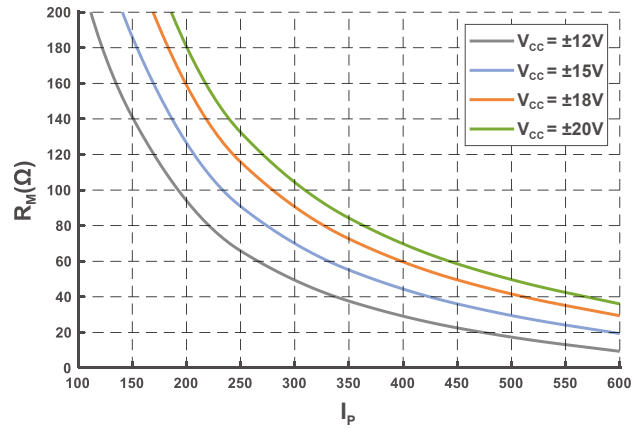
图 2 测量电阻 (@ T_A = 85\text{ }^\circ\text{C} )
