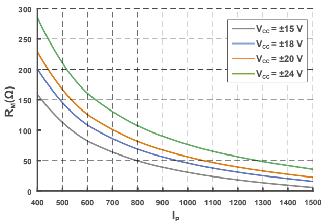
图 5 测量电阻 (@ T_A = 25\text{ }^\circ\text{C} )
