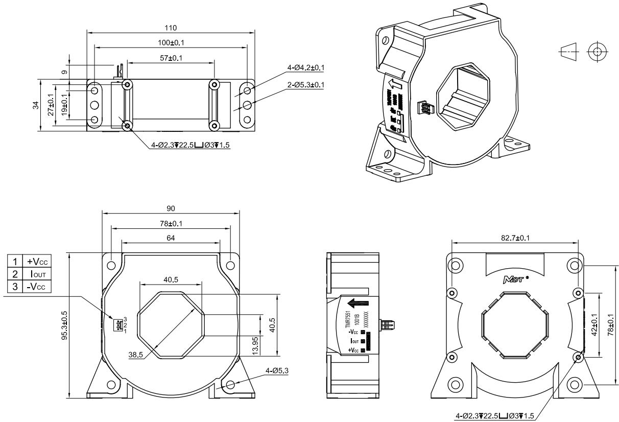
图 13 外形尺寸图（尺寸单位：mm）
