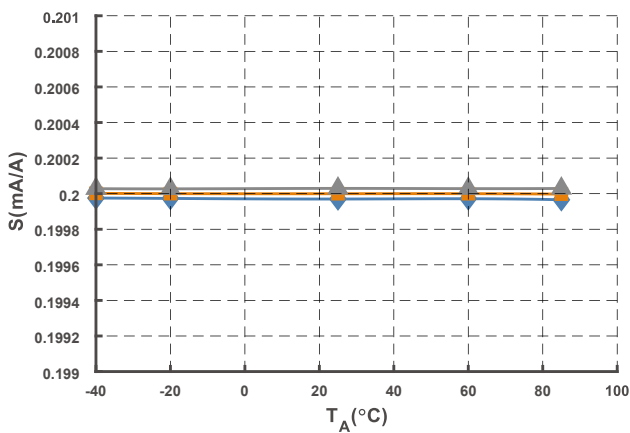
图10 灵敏度曲线
