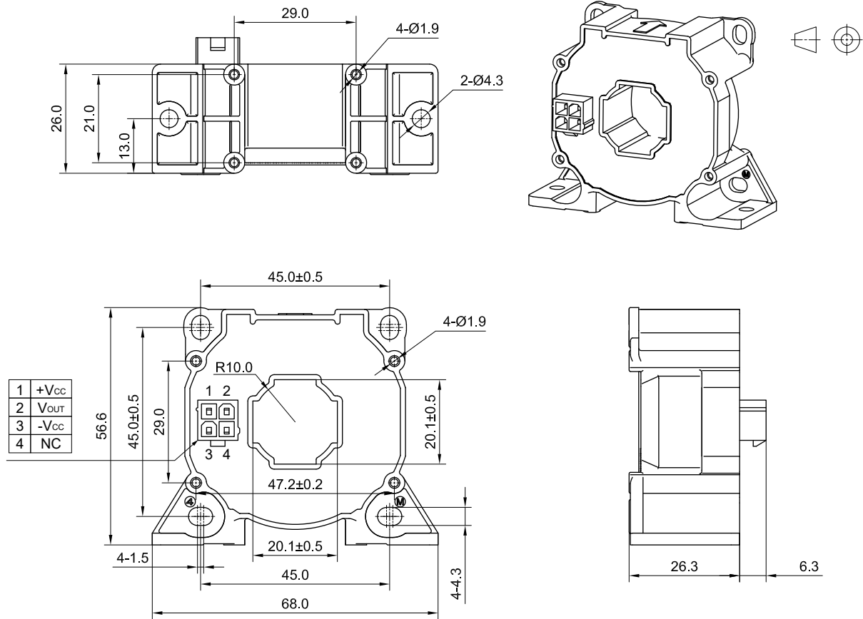
图 13 外形尺寸图 (尺寸单位: mm)
