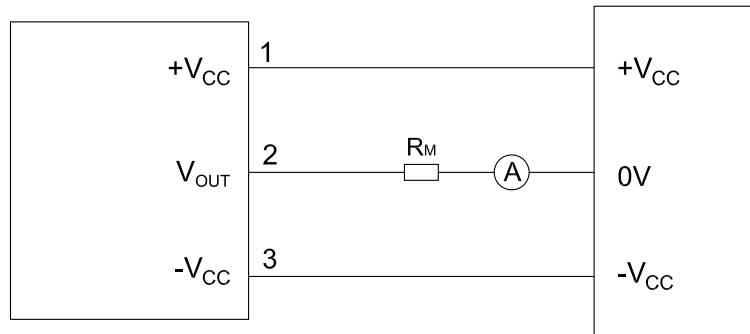
图 12 电气接口接线图
