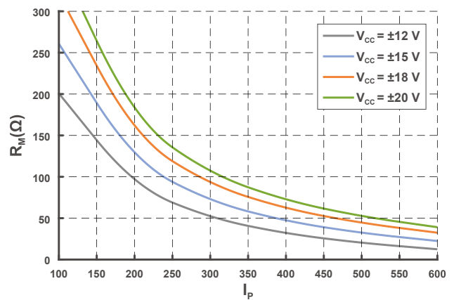
图 4 测量电阻 (@T A = 50 °C)
