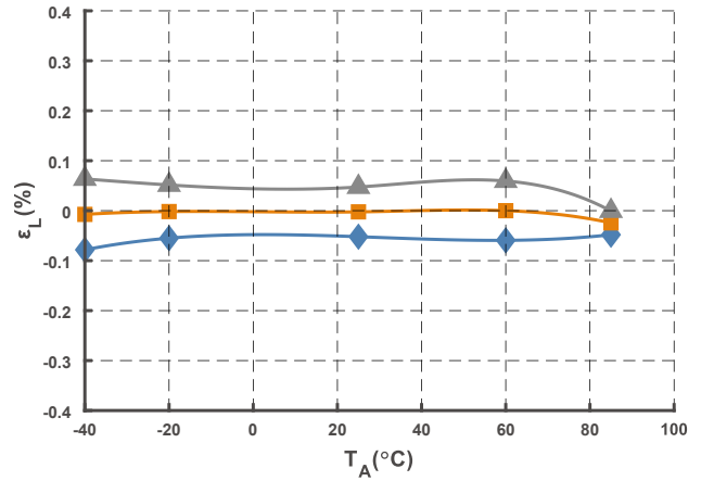
图 7 线性度曲线
