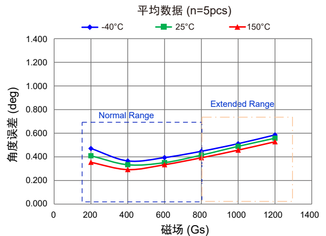
图 6 角度磁场曲线图
