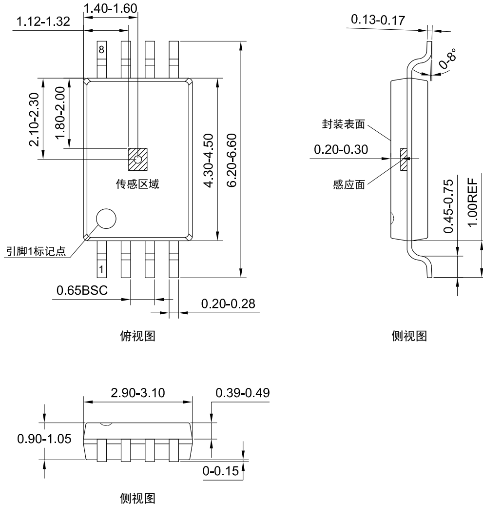
图 7 TSSOP8 封装图 (尺寸单位: mm)
