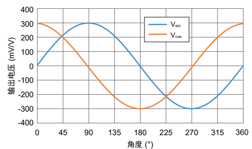
TMR3081 输出曲线
