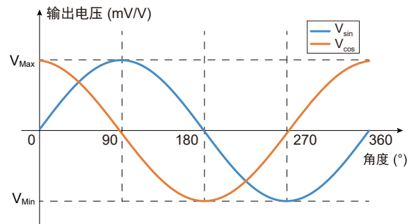
图 5 输出曲线
