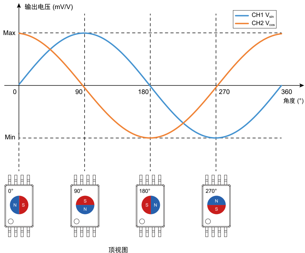
图 4 输出信号与磁铁关系示意图
