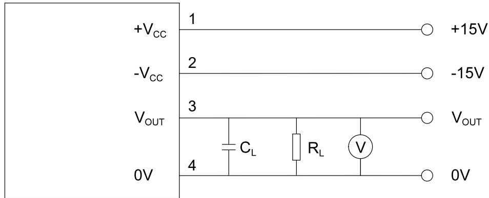
图 17 电气接口接线图
