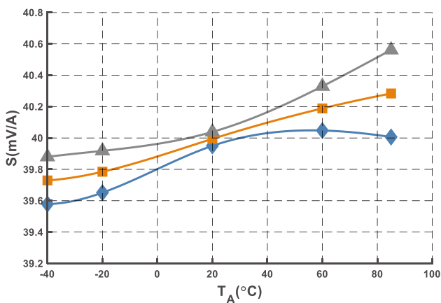
图10 灵敏度曲线 (@I PN = 100 A)
