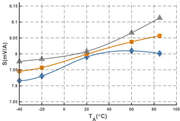
图 14 灵敏度曲线 (@I PN = 500 A)
