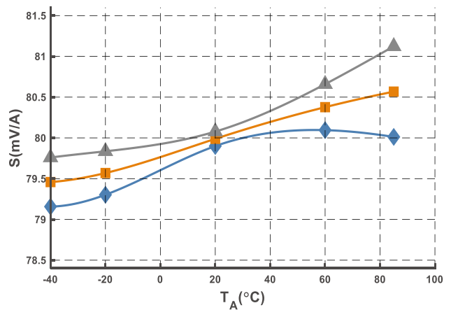
图9 灵敏度曲线 (@I PN = 50 A)
