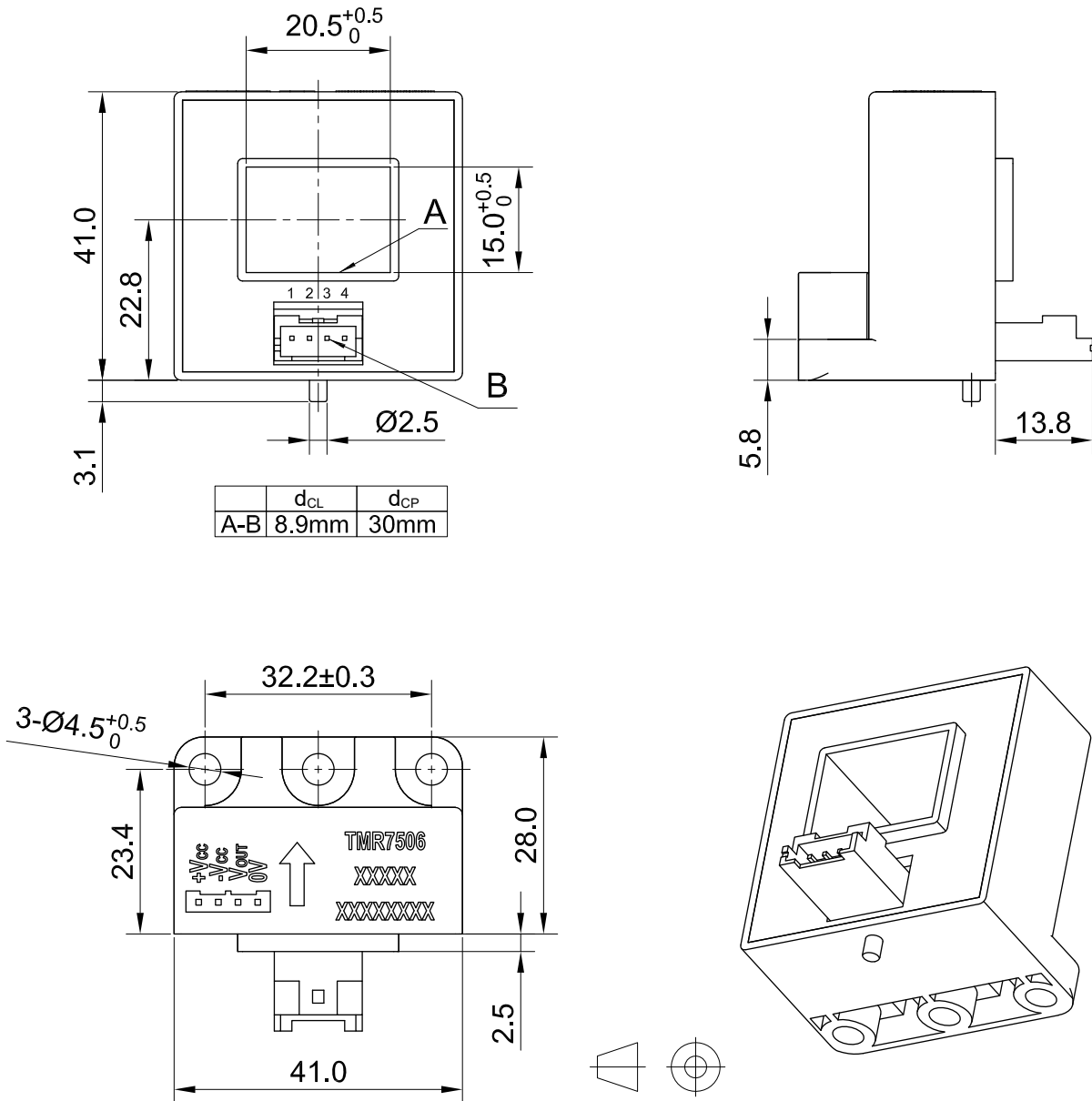
图 18 外形尺寸图（尺寸单位：mm）
