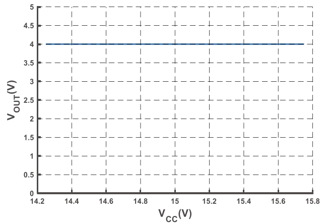
图 2 输出特性与供电电压曲线 (@ I_P = I_{PN} )
