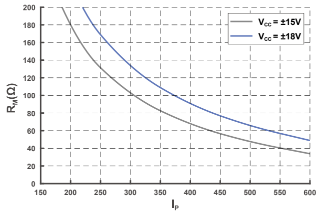
图 4 测量电阻 (@T A = 50 °C)
