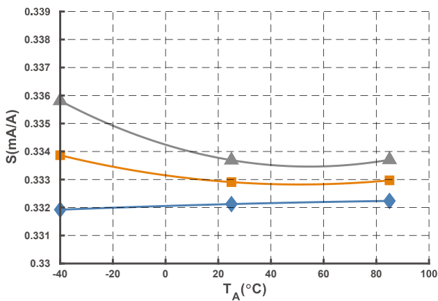
图 11 灵敏度曲线
