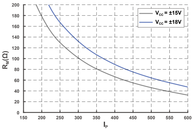
图 3 测量电阻 (@T A = 70 °C)
