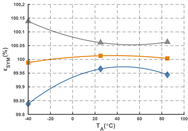
图 9 增益对称性曲线
