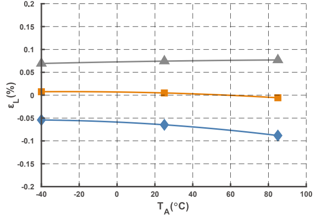
图 8 线性度曲线
