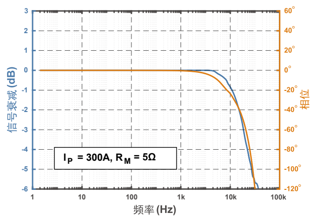
图 6 频响特性曲线
