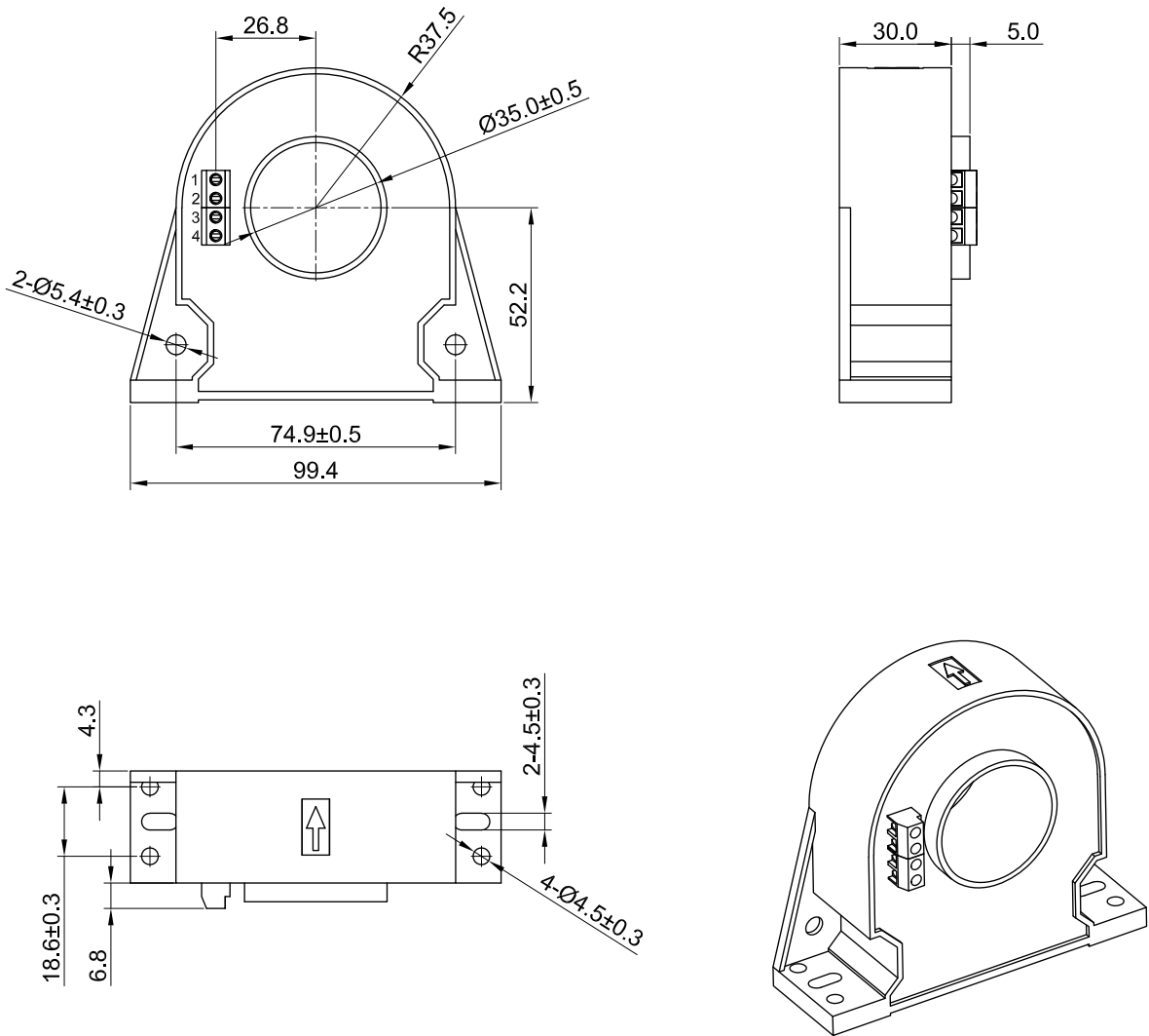
图 14 外形尺寸图（尺寸单位：mm）
