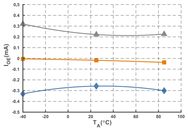
图 10 零点失调电流曲线
