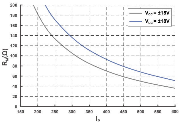
图 5 测量电阻 (@T A = 25 °C)
