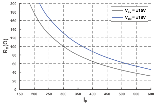
图 2 测量电阻 (@T A = 85 °C)
