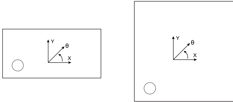
图 4-1 敏感方向 (DFN4L)
