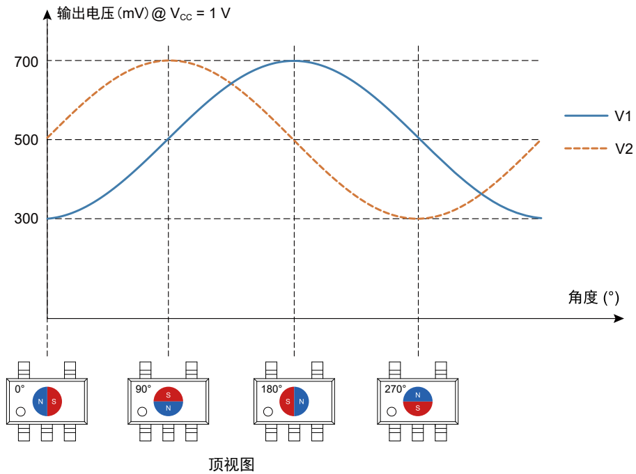
图 5-3 TMR3017S 输出信号与磁铁关系示意图
