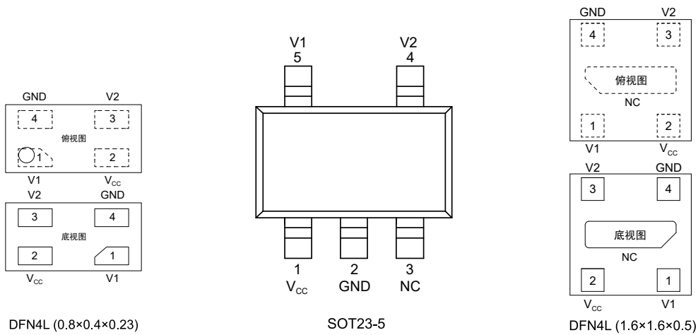
图 2 引脚定义
