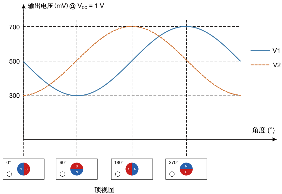
图 5-1 TMR3017D 输出信号与磁铁关系示意图
