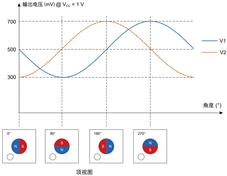
图 5-2 TMR3017BF 输出信号与磁铁关系示意图
