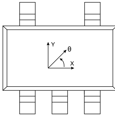
图 4-2 敏感方向 (SOT23-5)
