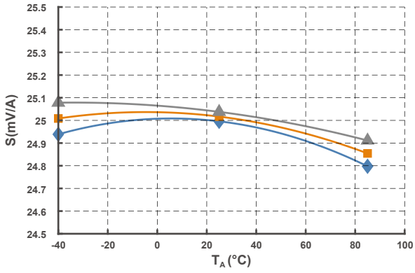
图 12 灵敏度曲线 (@I PN = 25 A)
