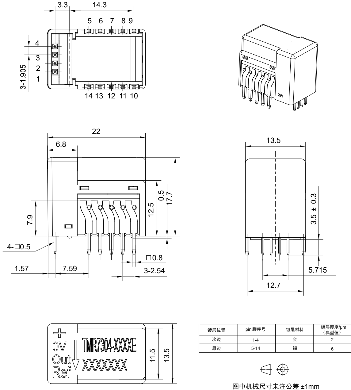
图 23 TMR7304-E 外形尺寸图 (尺寸单位: mm)
