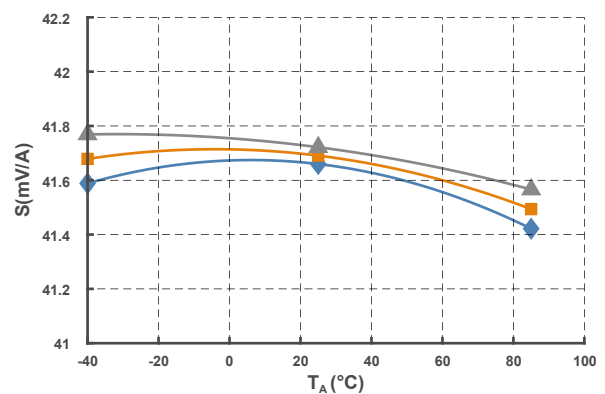
图 11 灵敏度曲线 (@I PN = 15 A)
