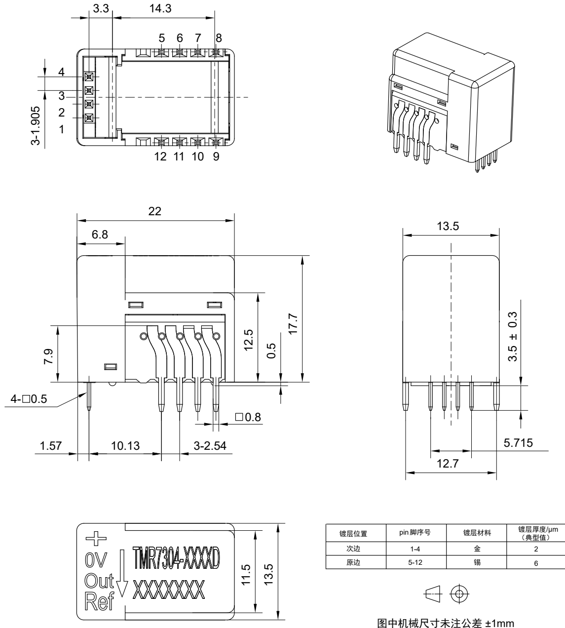
图 22 TMR7304-D 外形尺寸图 (尺寸单位: mm)
