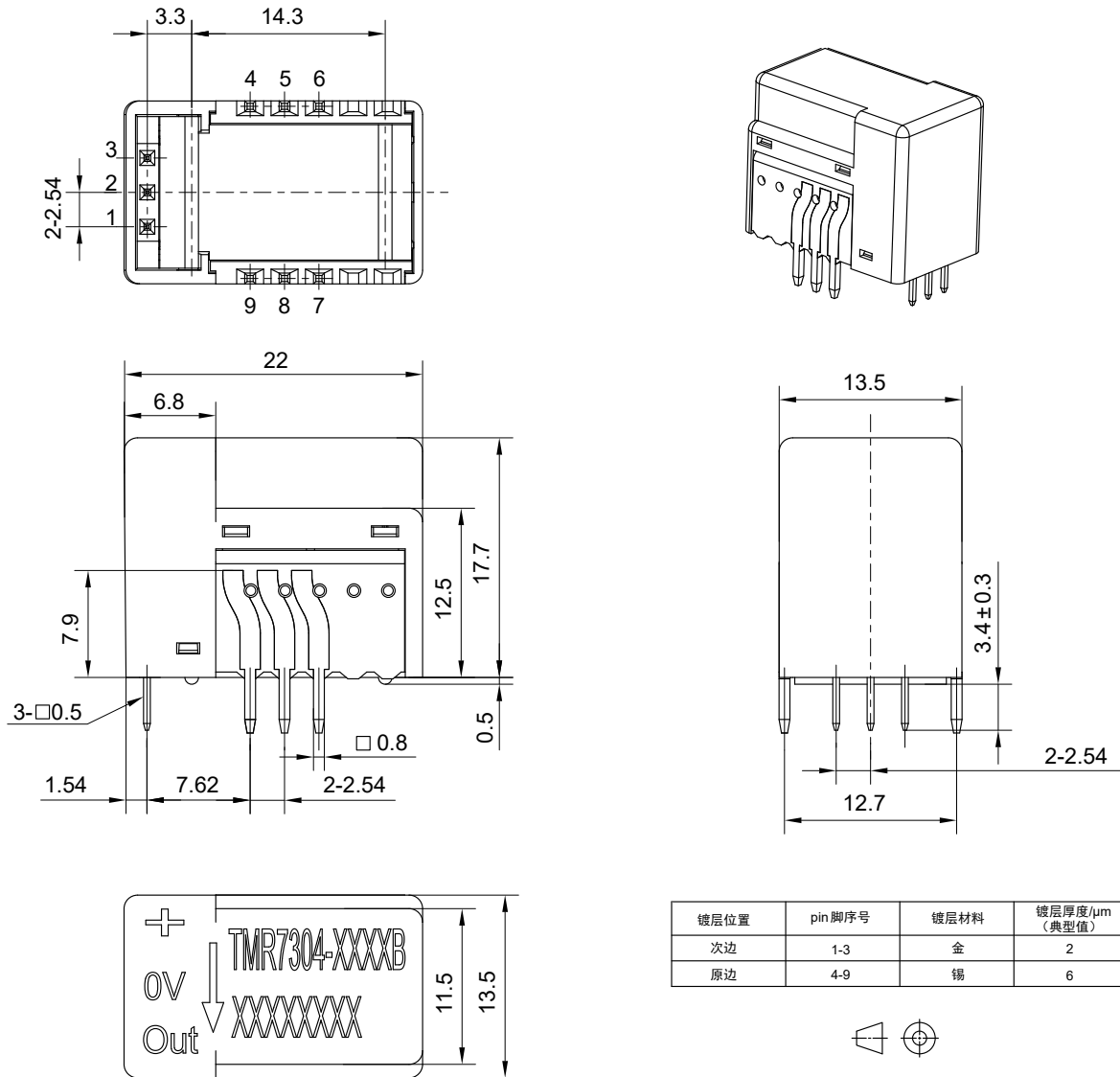
TMR7304-B 外形尺寸图
