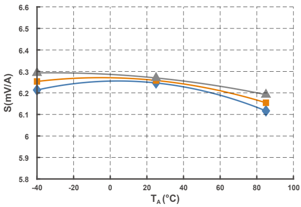
图 14 灵敏度曲线 (@I PN = 75 A)
