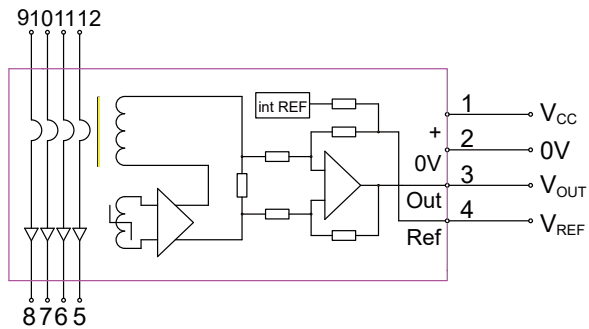
图 18 TMR7304-D 电气连接图
