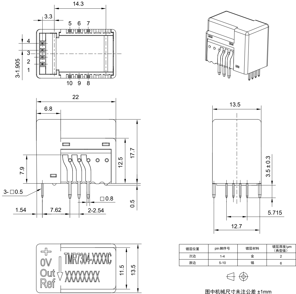
图 21 TMR7304-C 外形尺寸图 (尺寸单位: mm)
