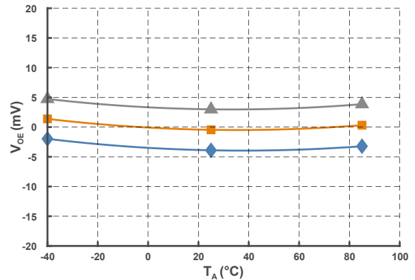
图 9 零点失调电压曲线
