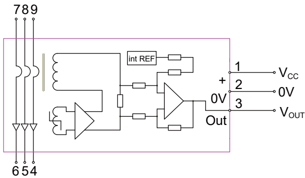
图 16 TMR7304-B 电气连接图
