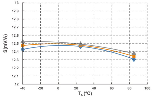
图 13 灵敏度曲线 (@I PN = 50 A)
