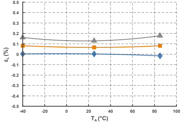
图 7 线性度曲线
