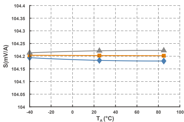
图 10 灵敏度曲线 (@I PN = 6 A)
