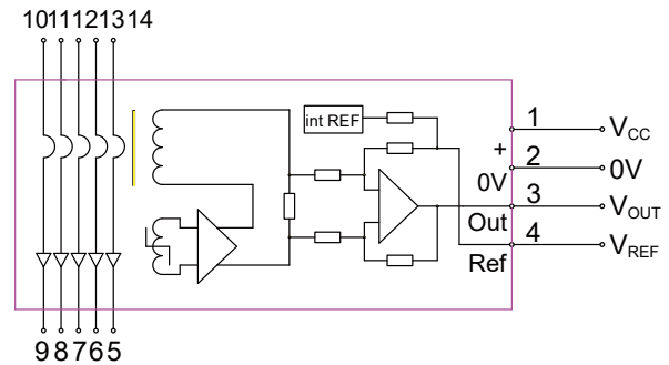
图 19 TMR7304-E 电气连接图
