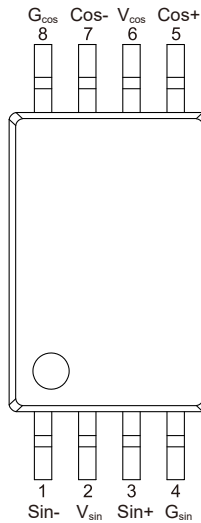
图 2 引脚定义
