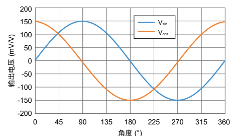
TMR3083 输出曲线
