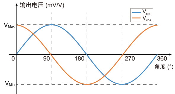
图 5 输出曲线
