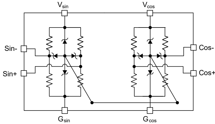
图 1 芯片内部原理框图
