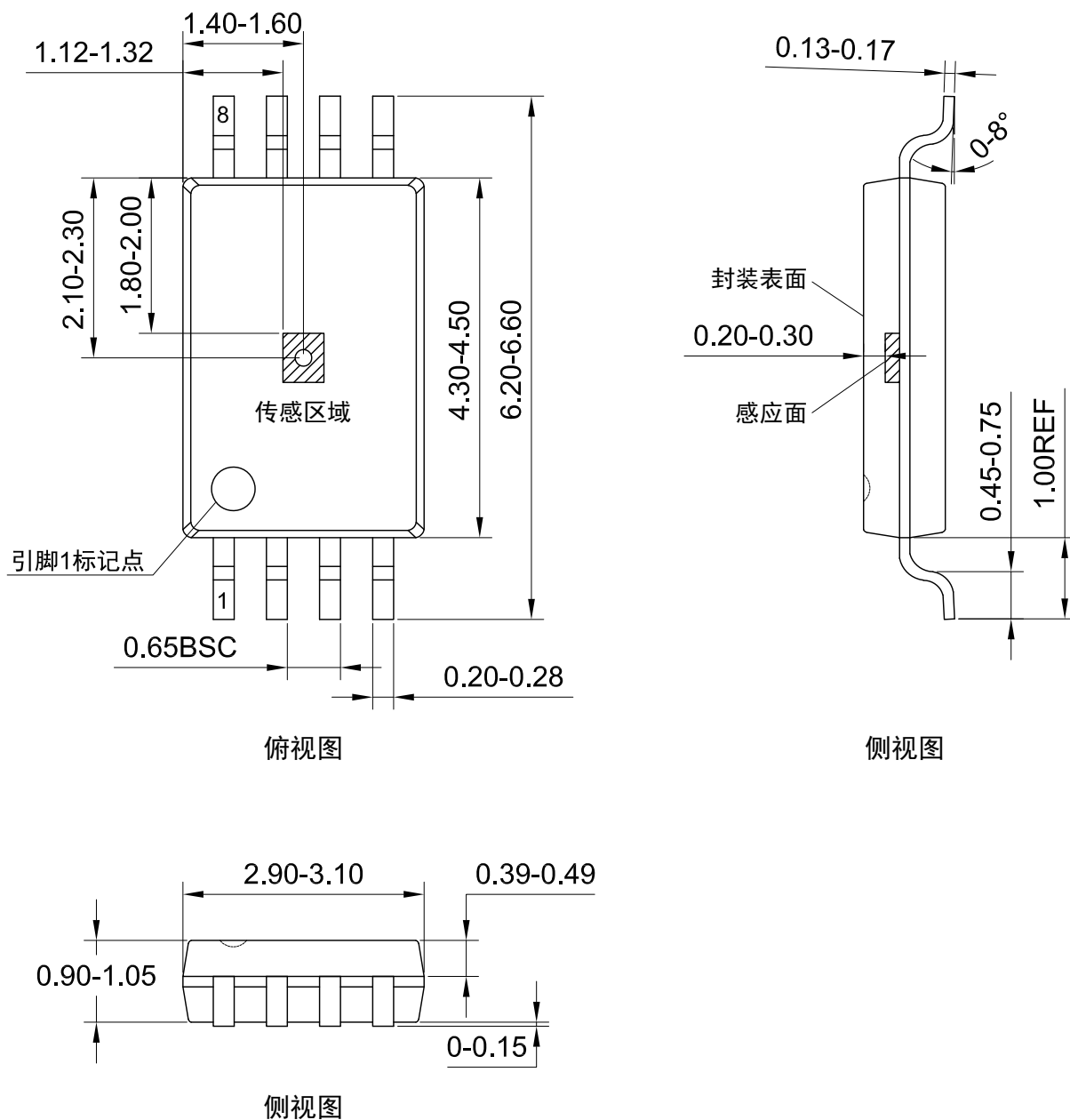
图 6 TSSOP8 封装图 (尺寸单位: mm)
