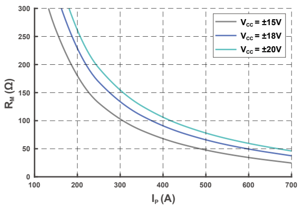
图 5 测量电阻 (@T A = 50 °C)
