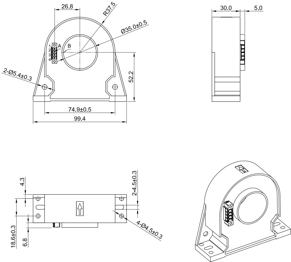
图 8 外形尺寸图（尺寸单位：mm）
