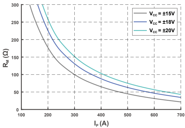
图 3 测量电阻 (@T A = 85 °C)
