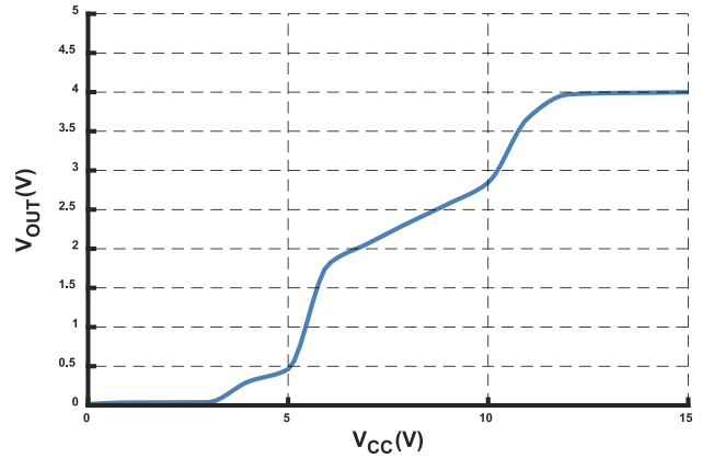
图 2 输出特性与供电电压曲线 (@ I_P = I_{PN} )
