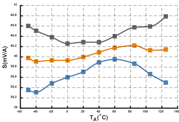
图10 灵敏度曲线 (@ I_{PN} = 100\text{ A} )
