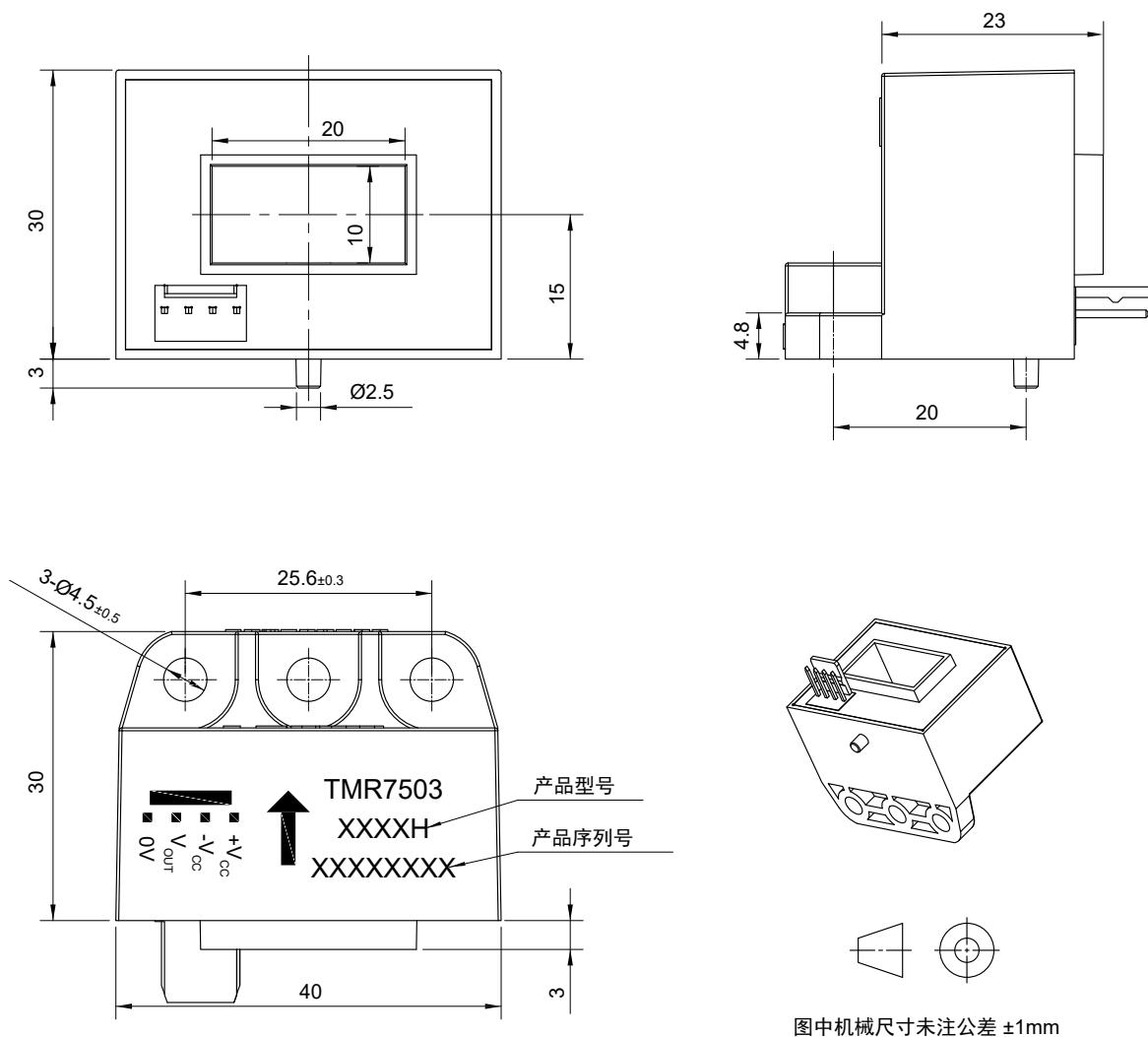
图 18 外形尺寸图 (尺寸单位: mm)
