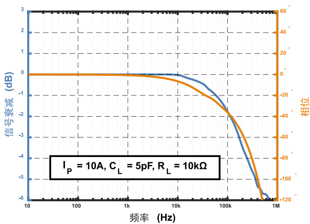
图 5 频响特性曲线
