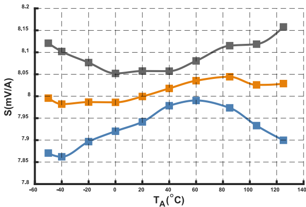
图 14 灵敏度曲线 (@ I_{PN} = 500\text{ A} )
