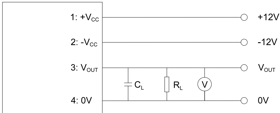
图 17 电气接口接线图
