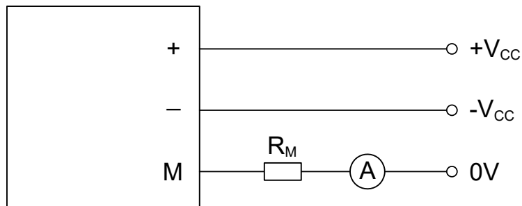
图 1 电气接口接线图
