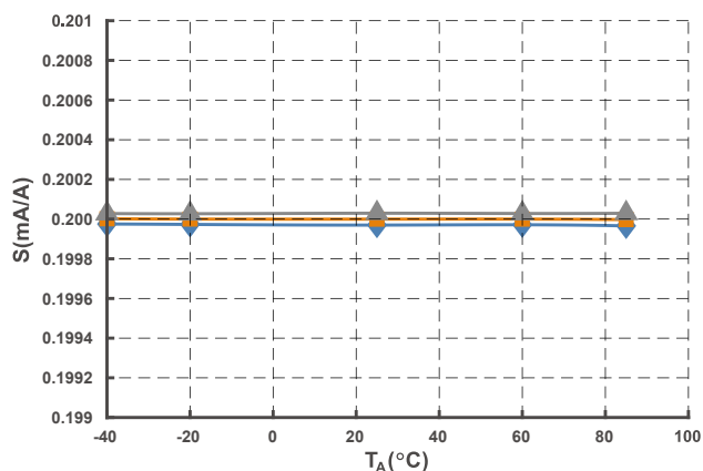
图 10 灵敏度曲线
