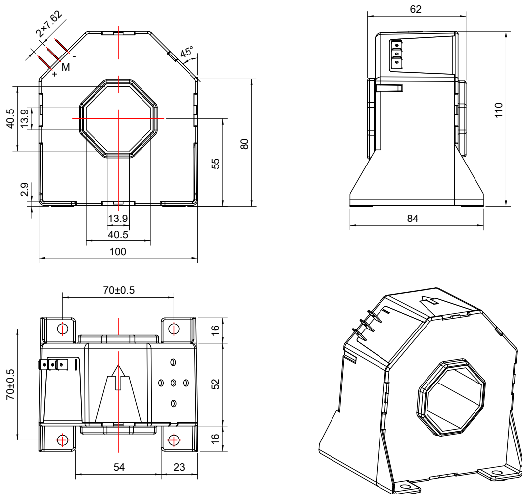
图 13 外形尺寸图（尺寸单位：mm）
