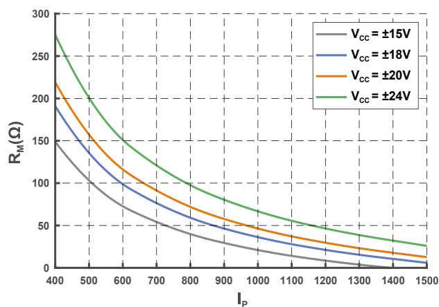
图 2 测量电阻 (@ T_A = 85^\circ C )
