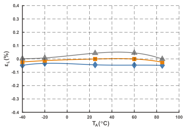
图 7 线性度曲线
