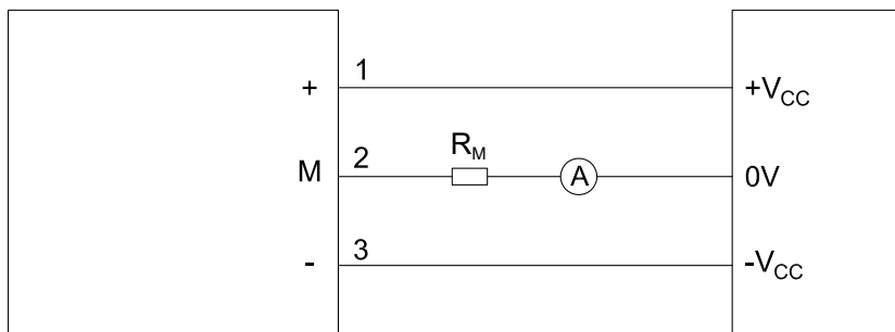
图 12 电气接口接线图
