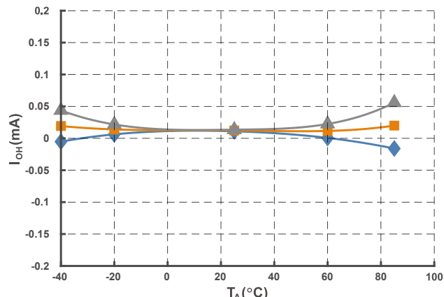
图 11 磁滞特性曲线
